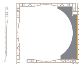
cajón con aislante: Neopor + masa pesada.
