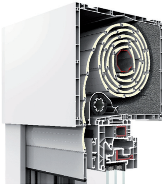
cajón DE 200mm con MOSQUITERA INTEGRADA.
