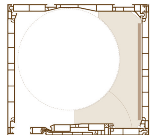
cajón 190 mm
