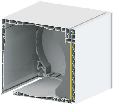
cajón con aislante: Neopor + masa pesada.
